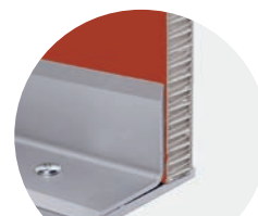
SYSTÈME GRIP. Pince ajustable par glissement et serrage
